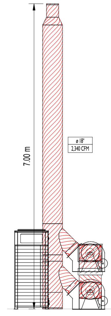
4 Extraccion BLSL2 1 : 50
