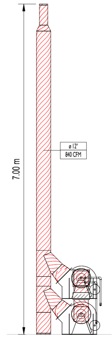
3 Extraccion BSL3 1 : 50
